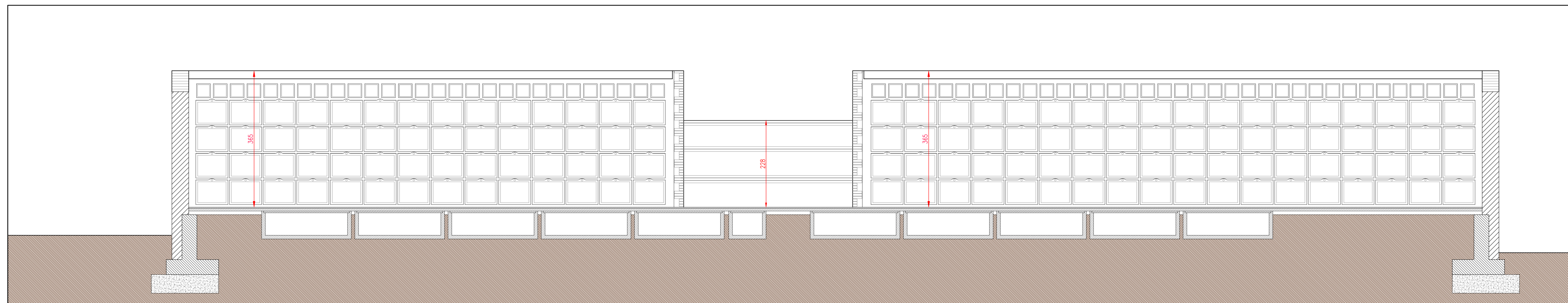
SEZIONE B'-B'
